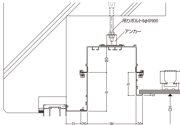
吊ボルトによる納まり例(天井上がり)
