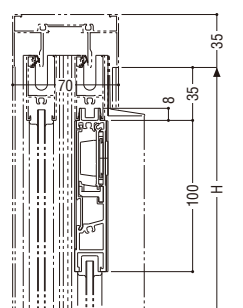
(ガラス溝幅14mm)
