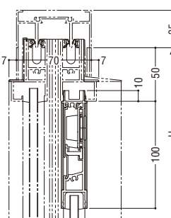
(ガラス溝幅20mm)
