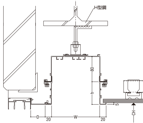
吊ボルトによる納まり例(天井上がり)
