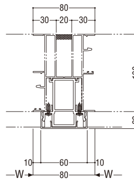
KA方立
