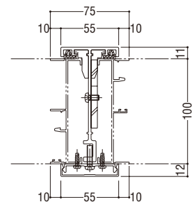
A1方立
