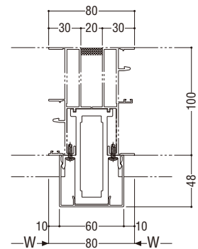
KB方立
