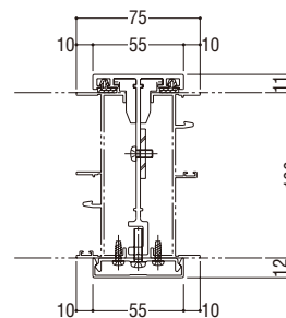
A方立
