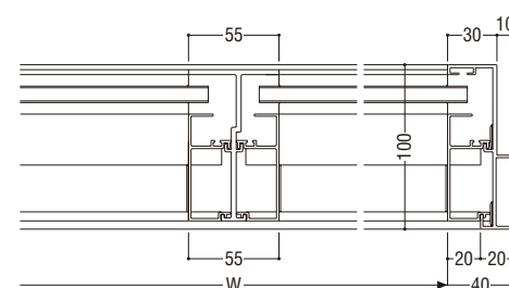
中間方立①
