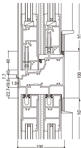
6 インペイ外倒し排煙 / 引違い
