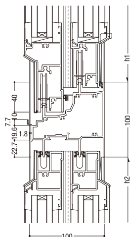
8 インペイ外倒し排煙 / 引違い
