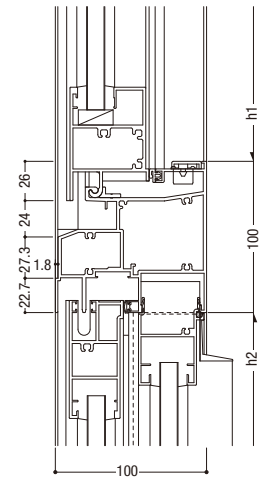
21 FIX／外動片引き
