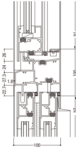
5 外倒し排煙／外動片引き
