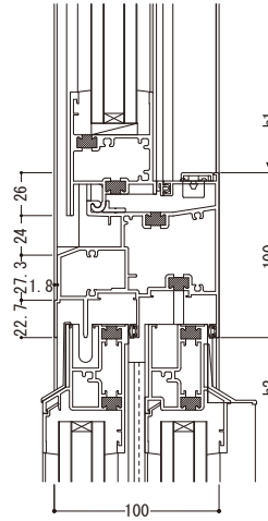
7 外倒し排煙／両袖可動
