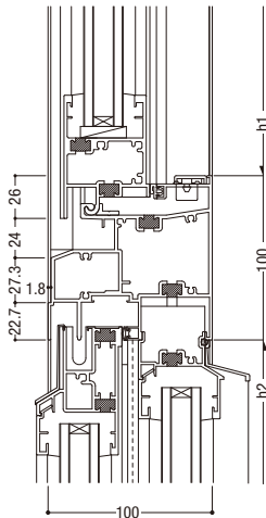
9 外倒し排煙／両袖可動
