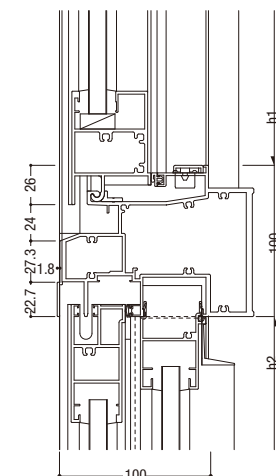
33 FIX／両袖可動
