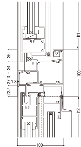
22 FIX／外動片引き
