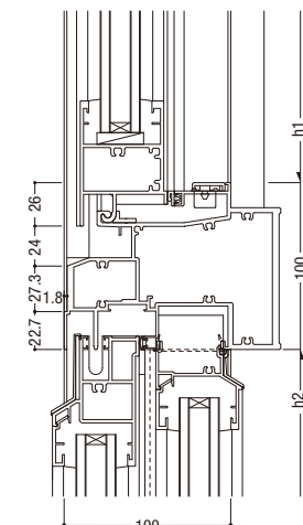
35 FIX／両袖可動
