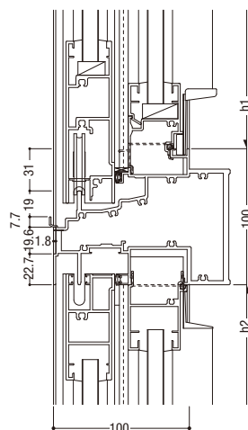
29 インペイ外倒し排煙／両袖可動
