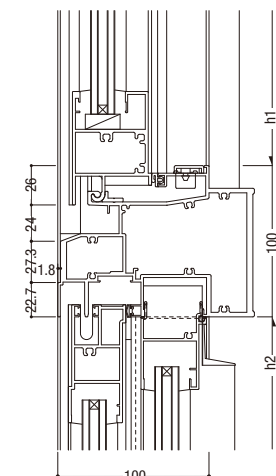
34 FIX／両袖可動
