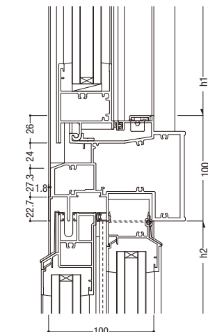
36 FIX／両袖可動
