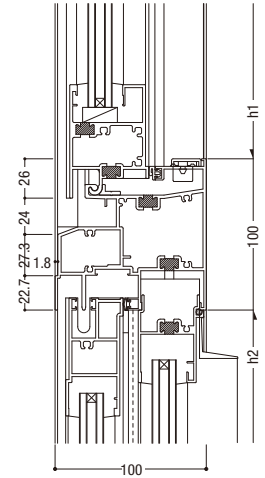
8 外倒し排煙／両袖可動
