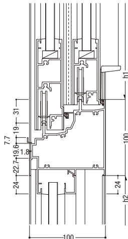
45 外動片引き / FIX
