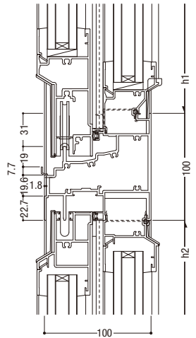
20 インペイ外倒し排煙／外動片引き
