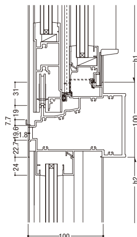
54 外開き / FIX たてすべり出し / FIX
