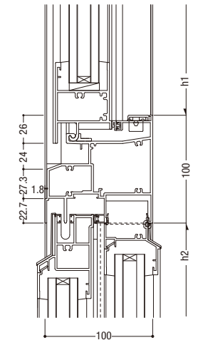
24 FIX／外動片引き
