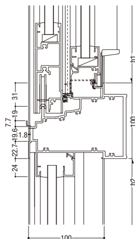
53 外開き / FIX たてすべり出し / FIX
