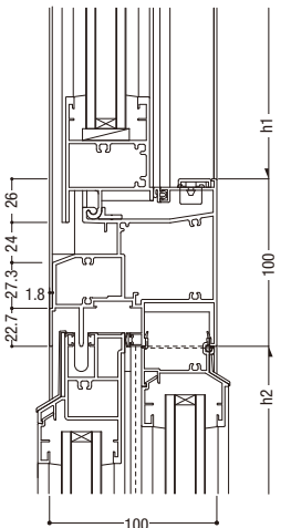
23 FIX／外動片引き
