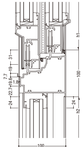
48 外動片引き / FIX
