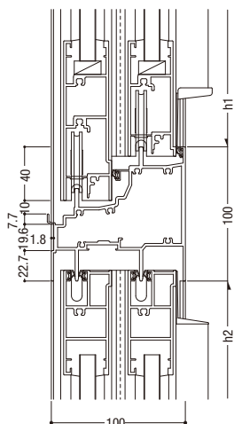
5 インペイ外倒し排煙 / 引違い
