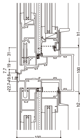
30 インペイ外倒し排煙／両袖可動
