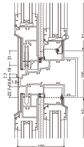
31 インペイ外倒し排煙／両袖可動
