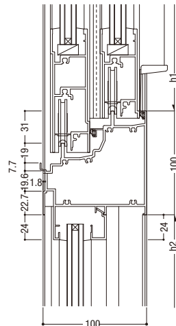
46 外動片引き / FIX
