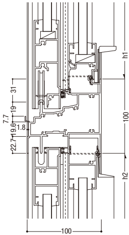
17 インペイ外倒し排煙／外動片引き
