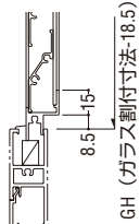
中骨納まりの場合
