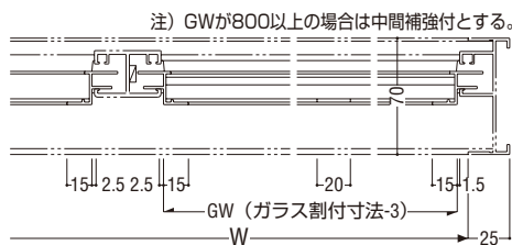
GH (ガラス割付寸法-9)
