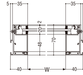
横断面図
