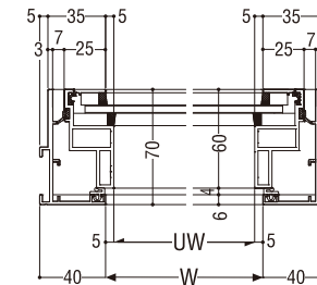
段窓横断面図
