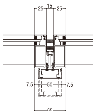
Fix窓-Fix窓
