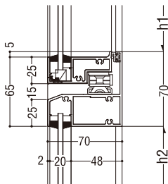
たて断面図
