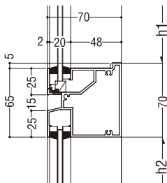
たて断面図
