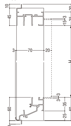
FIX部15
