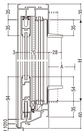
WDタイプ (FIX部20)
