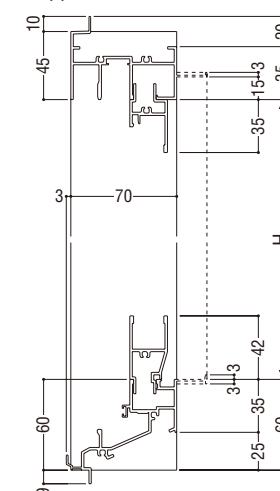
FIX部20
