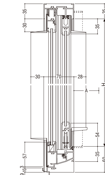
Dタイプ (FIX部15)
