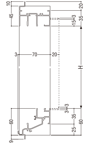
FIX部15
