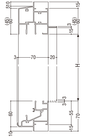
FIX部15
