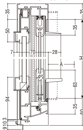
WEタイプ (FIX部20)
