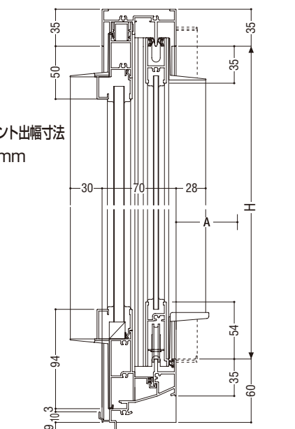
WDタイプ (FIX部20)
