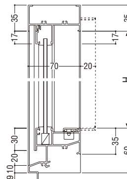
外押縁
