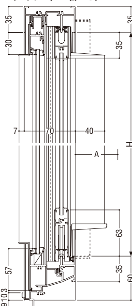
Eタイプ (FIX部15)
