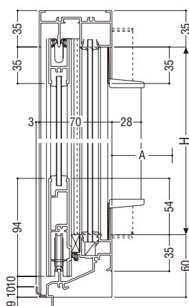
WDタイプ (FIX部20)
