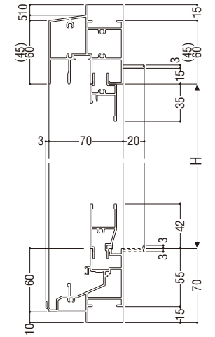
FIX部20
