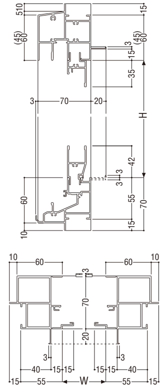
FIX部20
