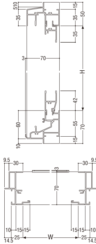
FIX部20
