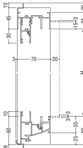
FIX部15
