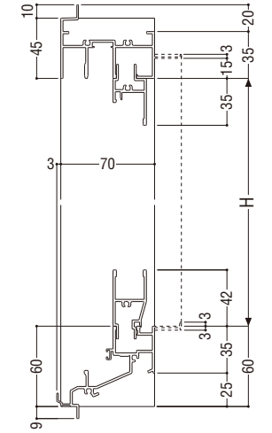
FIX部20
