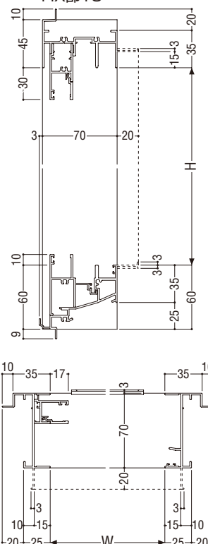
FIX部15
