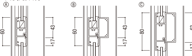
中骨(内押縁)
