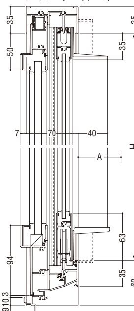
WEタイプ (FIX部20)
