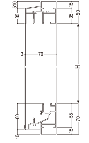
FIX部15
