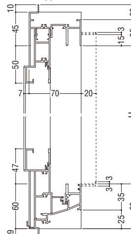
FIX部20
