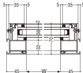
横断面図
