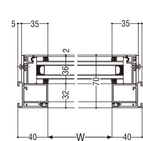
横断面図
