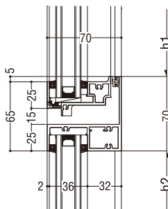
たて断面図
