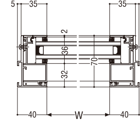
横断面図
