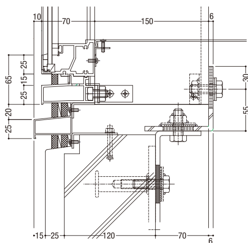
立ち上がり部
