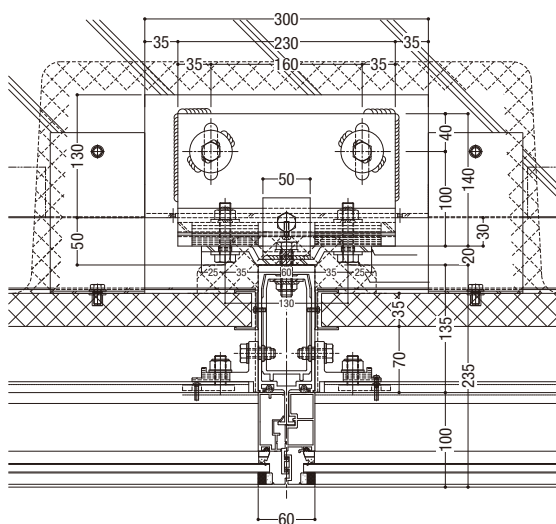
ファスナー・ブラケット詳細
