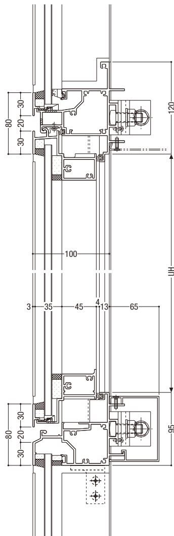
a—a 突き出し排煙窓
