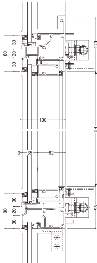
c—c 袖FIX窓
