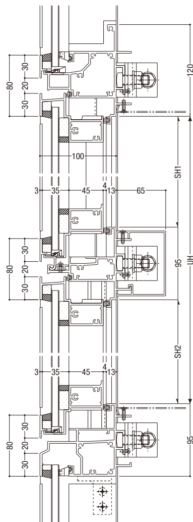
c—c 外倒し排煙窓/たてすべり出し窓
