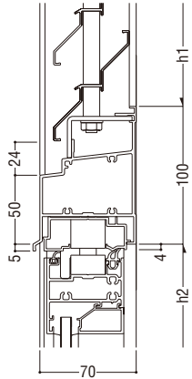
30 インペイ内倒し排煙 / 片開きドア・両開きドア
