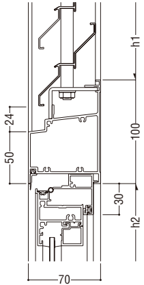
29 突出し排煙 (インペイと共通) / 片開きドア・両開きドア
